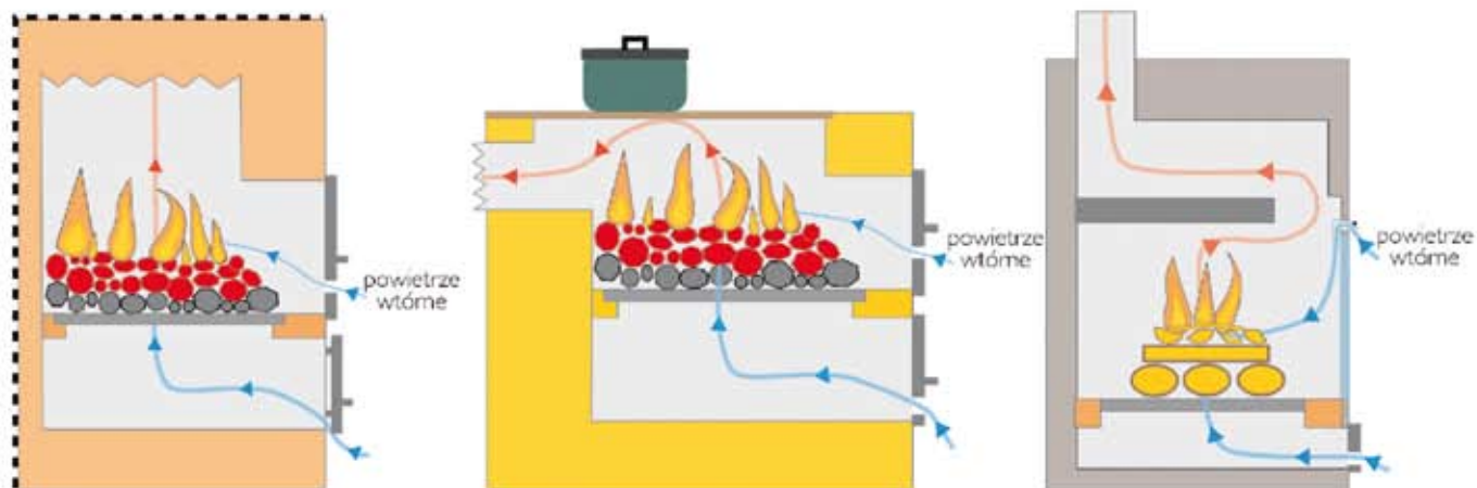
Piec kaflowy
